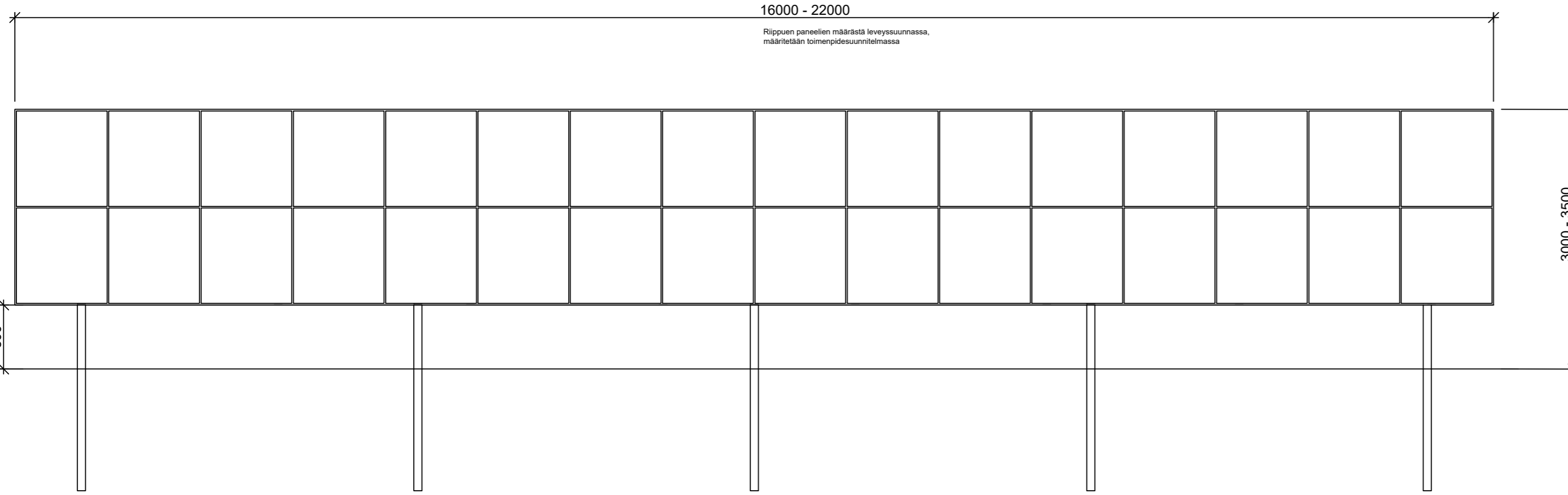
JULKISIVU
